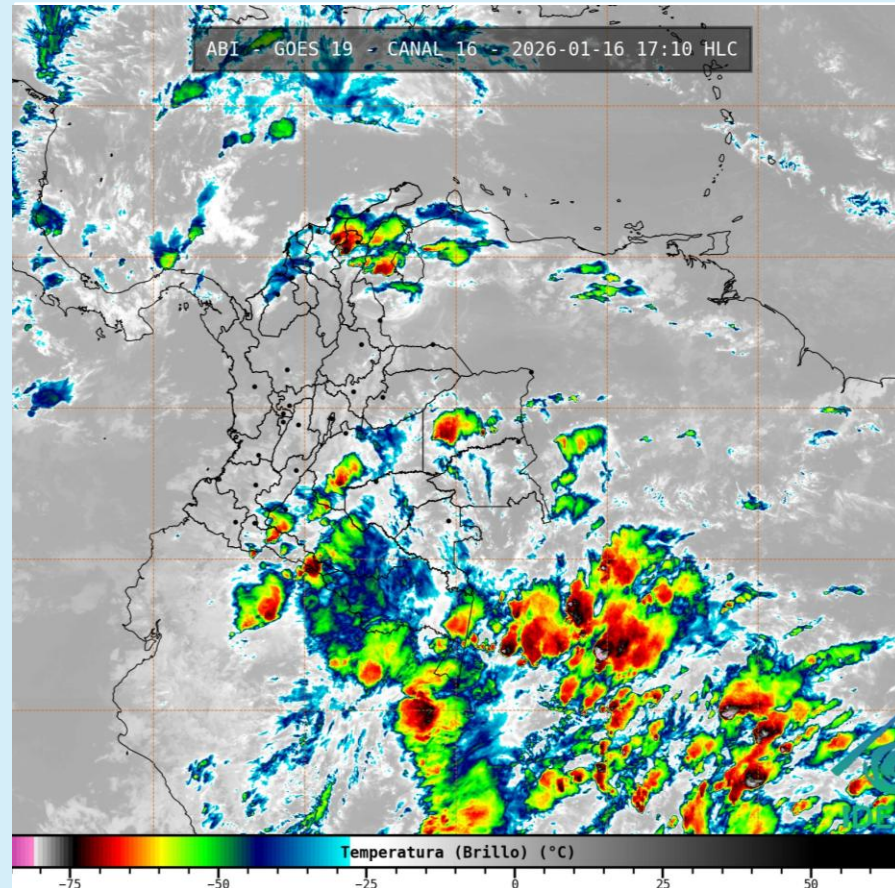
Imagen GOES 19 (East) Canal Infrarrojo 16 de enero de 2026– Hora 17:10 HLC Fuente: IDEAM - GOES 19
