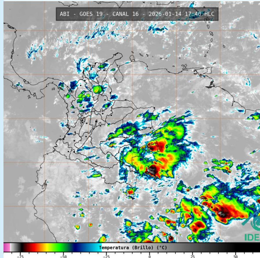
Imagen GOES 19 (East) Canal Infrarrojo 14 de enero de 2026– Hora 17:40 HLC Fuente: IDEAM - GOES 19
