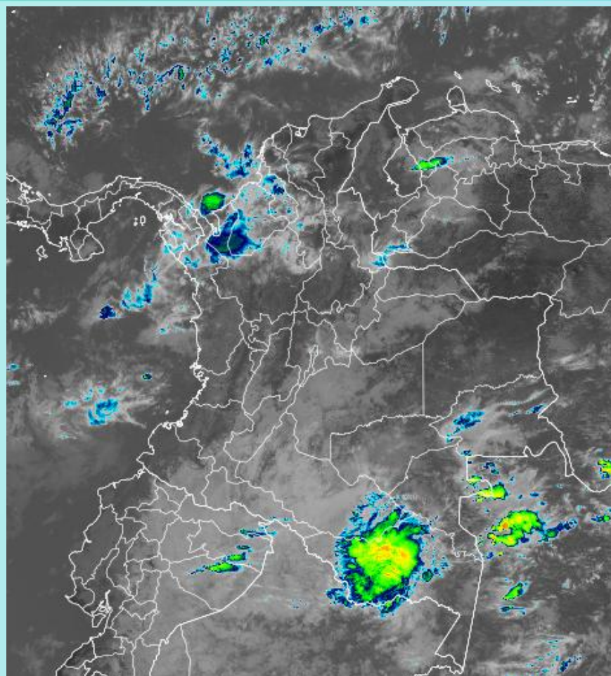
Imagen GOES 19 East Canal Infrarrojo, 14 de enero de 2026 - Hora 11:40 HLC. Fuente: https://bart.ideam.gov.co GOES 19
