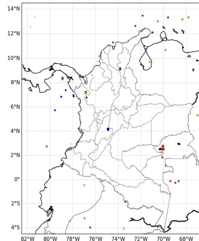
DESCARGAS ELÉCTRICAS GOES 19 MAPA NACIONAL
