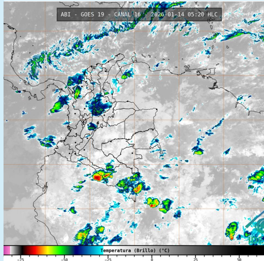
Imagen GOES 19 (East) Canal Infrarrojo 14 de enero de 2026– Hora 05:20 HLC Fuente: IDEAM - GOES 19
