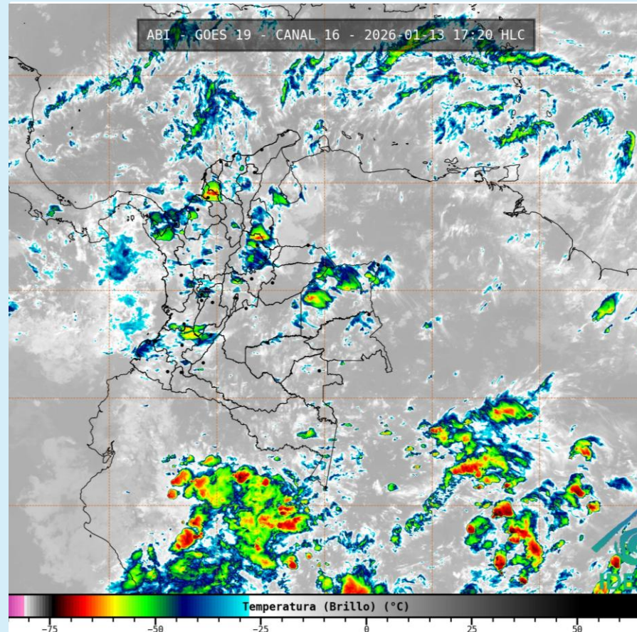
Imagen GOES 19 (East) Canal Infrarrojo 13 de enero de 2026– Hora 17:20 HLC Fuente: IDEAM - GOES 19
