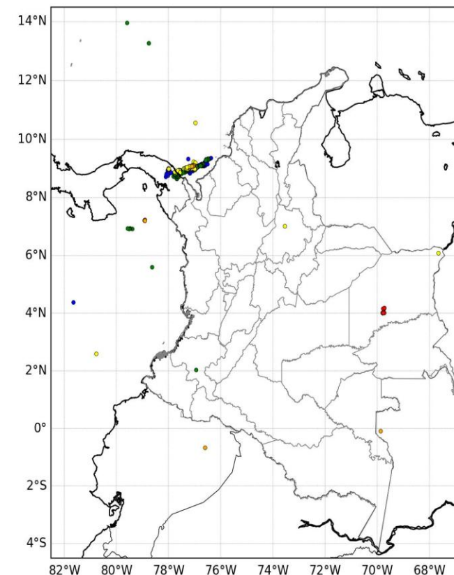
DESCARGAS ELÉCTRICAS GOES 19 MAPA NACIONAL
