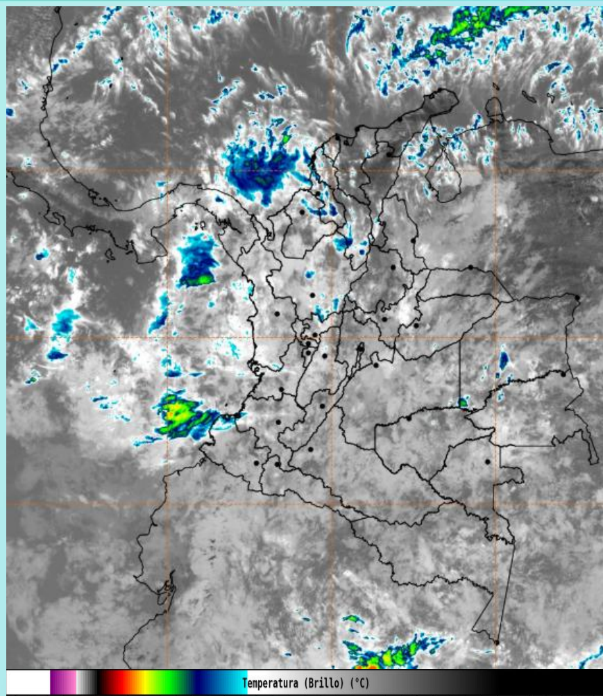
Imagen GOES 19 East Canal Infrarrojo, 13 de enero de 2026 - Hora 11:40 HLC. Fuente: https://bart.ideam.gov.co GOES 19
