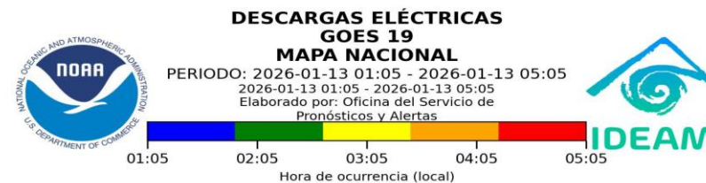
Descargas eléctricas (últimas horas) 13 de enero de 2026 – Hora entre las 01:05 - 05:05 HLC Fuente: IDEAM - NOAA
