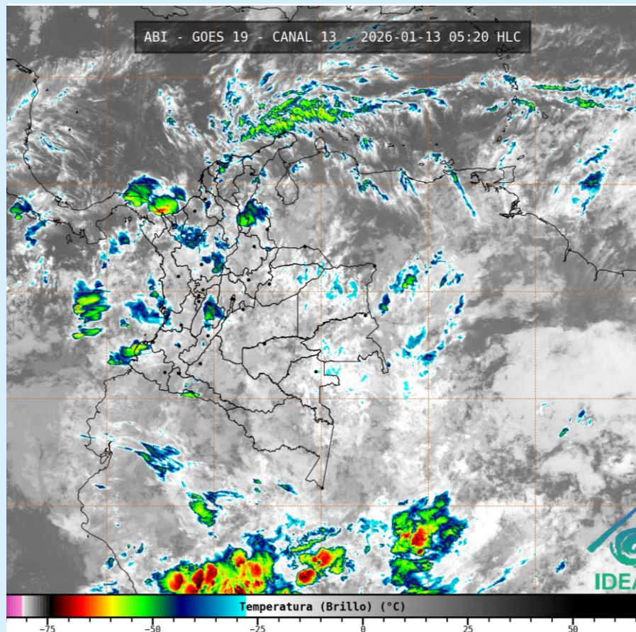
Imagen GOES 19 (East) Canal Infrarrojo 13 de enero de 2026– Hora 05:20 HLC Fuente: IDEAM - GOES 19
