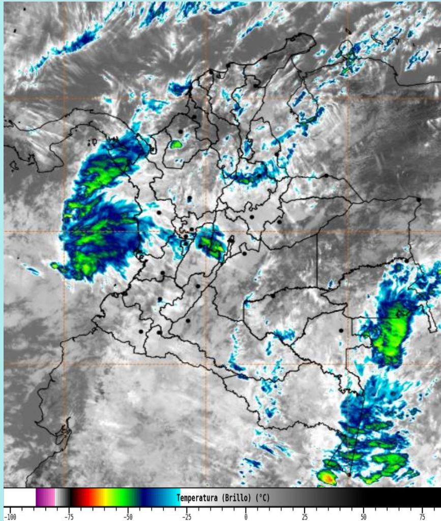
Imagen GOES 19 East Canal Infrarrojo, 12 de enero de 2026 - Hora 12:00 HLC. Fuente: https://bart.ideam.gov.co GOES 19
