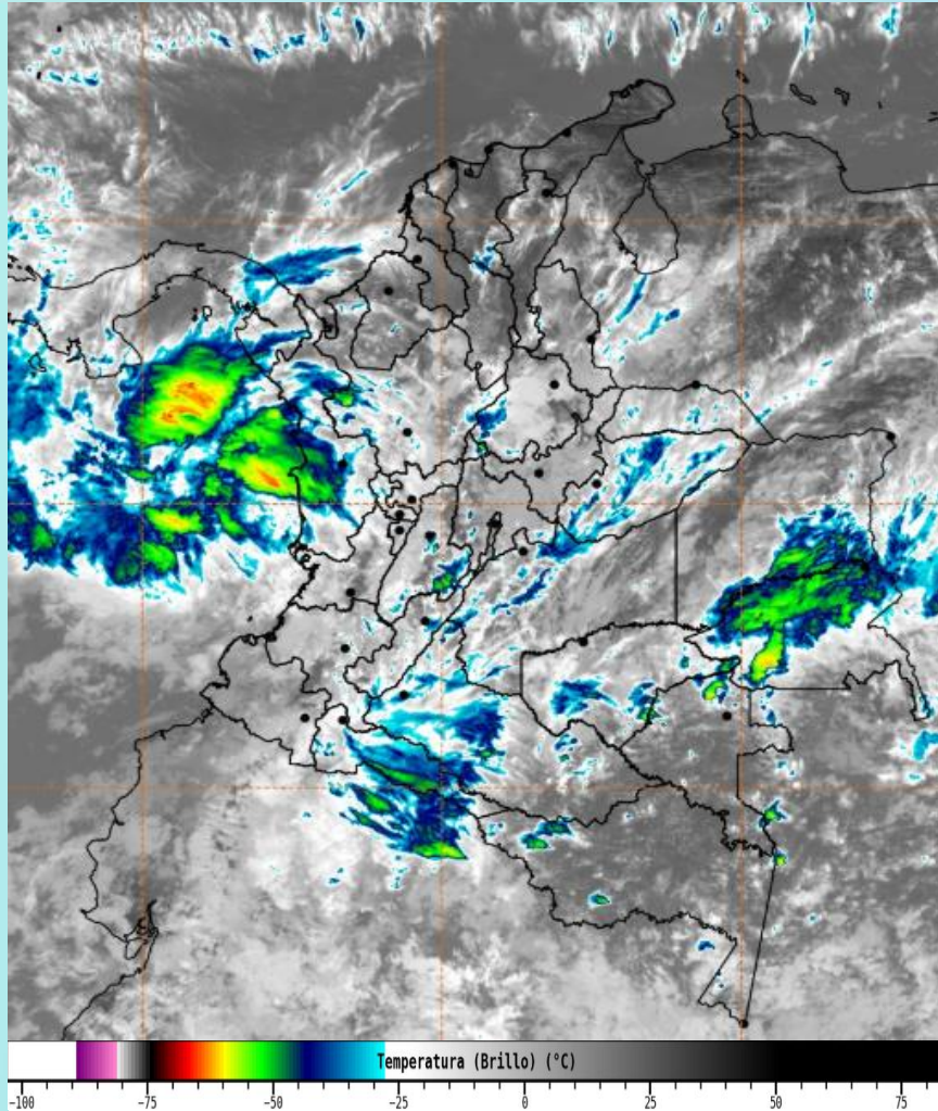
Imagen GOES 19 East Canal Infrarrojo, 11 de enero de 2026 - Hora 12:00 HLC. Fuente: https://bart.ideam.gov.co GOES 19
