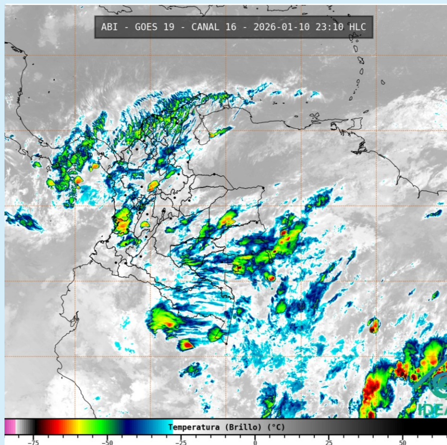
Imagen GOES 19 (East) Canal Infrarrojo 10 de enero de 2026– Hora 23:10 HLC Fuente: IDEAM - GOES 19
