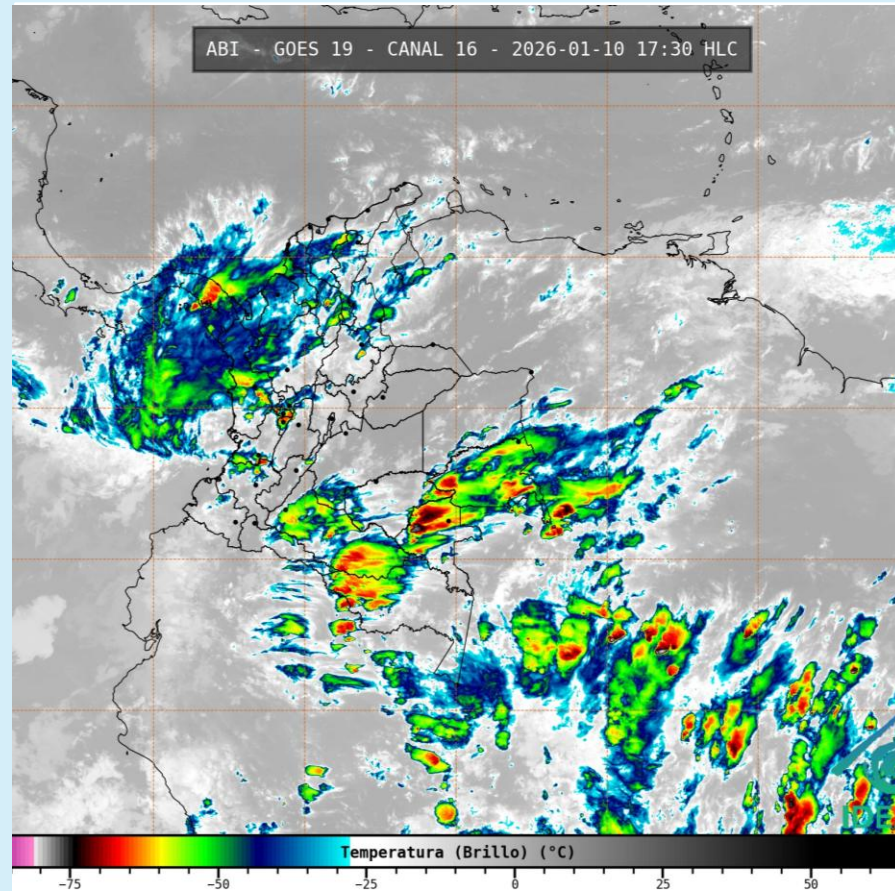
Imagen GOES 19 (East) Canal Infrarrojo 10 de enero de 2026– Hora 17:30 HLC Fuente: IDEAM - GOES 19
