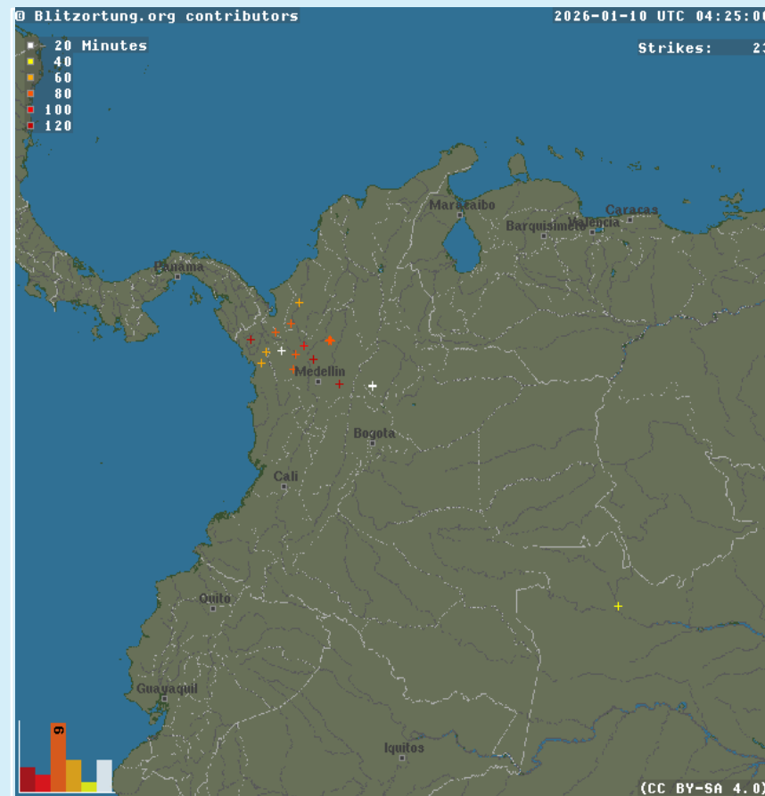
Descargas eléctricas (últimas horas) 9 de enero de 2026 – Hora 23:25 HLC Fuente: Blitzortung
