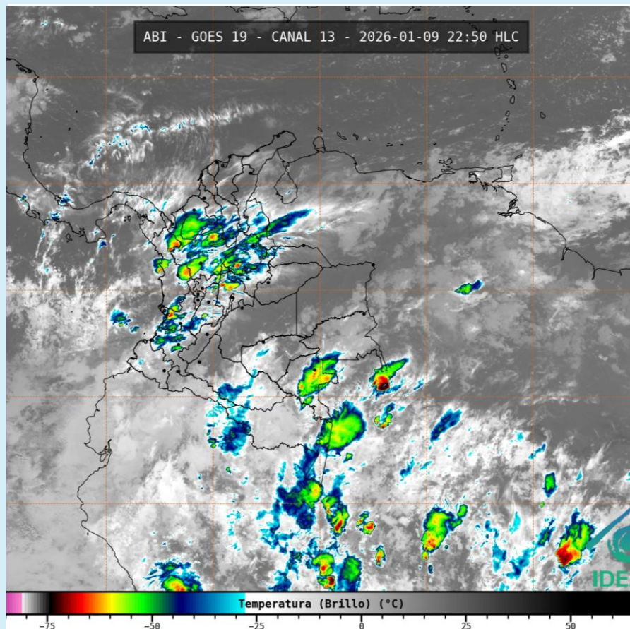
Imagen GOES 19 (East) Canal Infrarrojo 9 de enero de 2026– Hora 22:50 HLC Fuente: IDEAM - GOES 19
