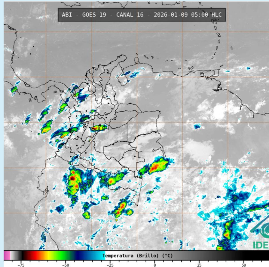
Imagen GOES 19 (East) Canal Infrarrojo 9 de enero de 2026– Hora 05:00 HLC Fuente: RAMMB - GOES 19
