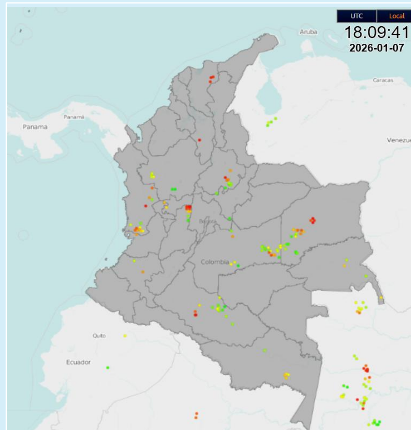
Descargas eléctricas (últimas tres horas) 7 de enero de 2026 – Hora 18:09 HLC Fuente: NOAA - IDEAM
