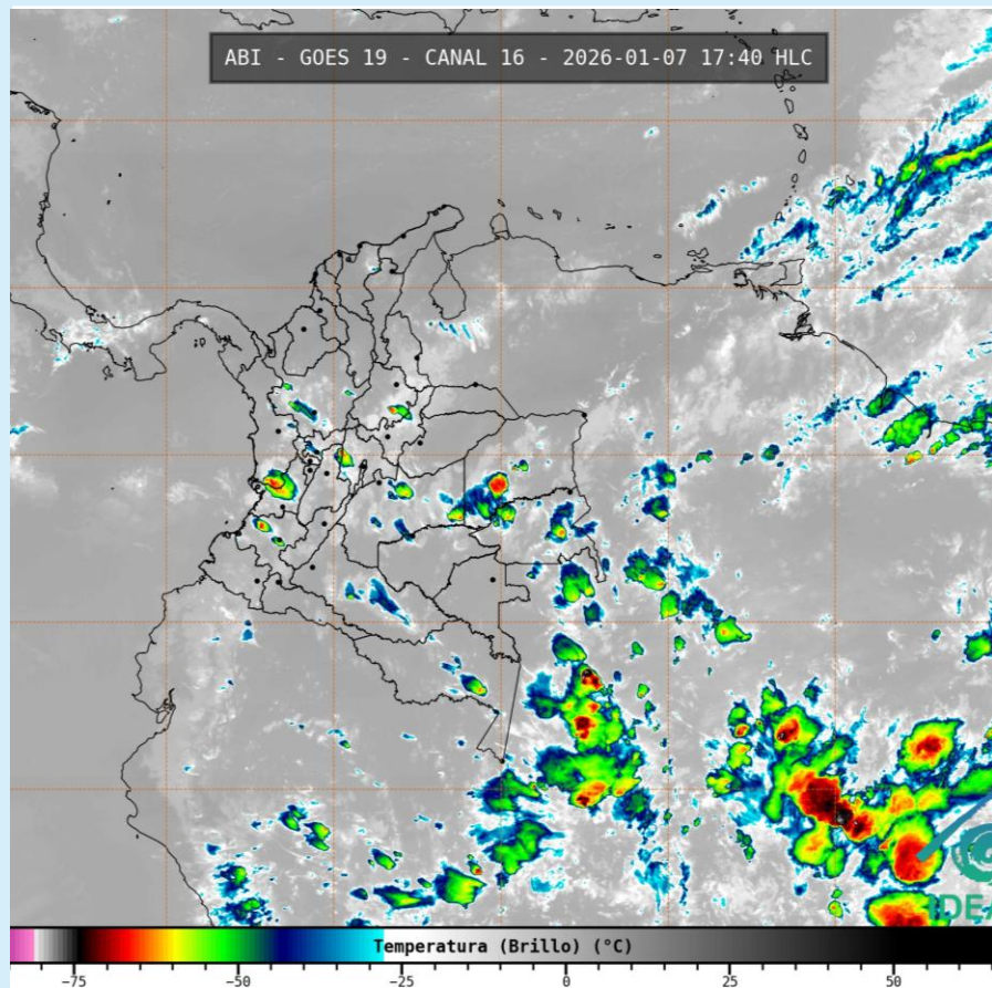
Imagen GOES 19 (East) Canal Infrarrojo 7 de enero de 2026– Hora 17:40 HLC Fuente: IDEAM - GOES 19
