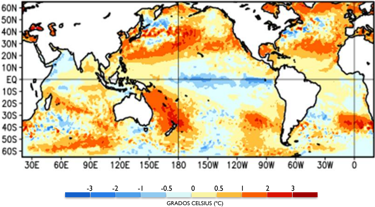
Promedio de las Anomalías de la Temperatura Superficial del Mar ( ^{\circ}\text{C} ) entre el 09 de noviembre y el 06 de diciembre de 2025. Fuente: NOAA
