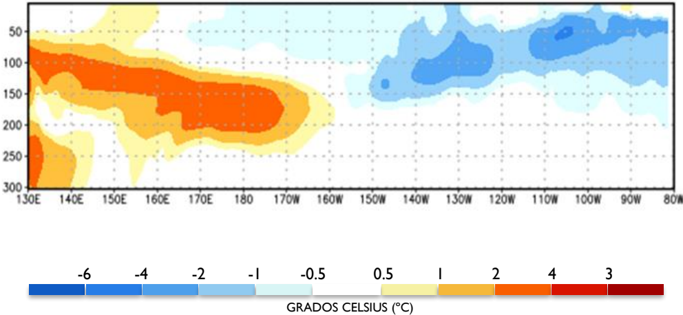
Anomalías de la Temperatura Subsuperficial del Mar ( ^{\circ}\text{C} ), pentada centrada en el 04 de diciembre 2025. Fuente: NOAA
