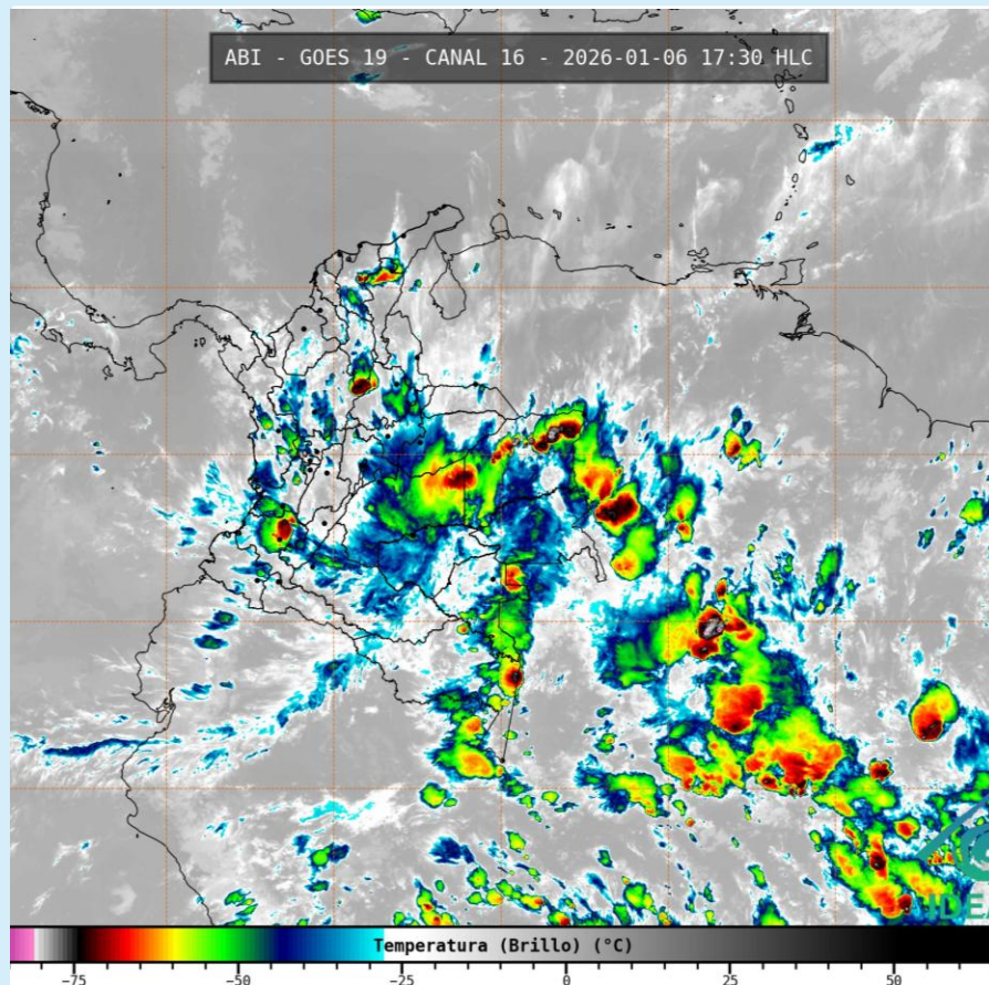
Imagen GOES 19 (East) Canal Infrarrojo 6 de enero de 2026– Hora 17:30 HLC Fuente: IDEAM - GOES 19
