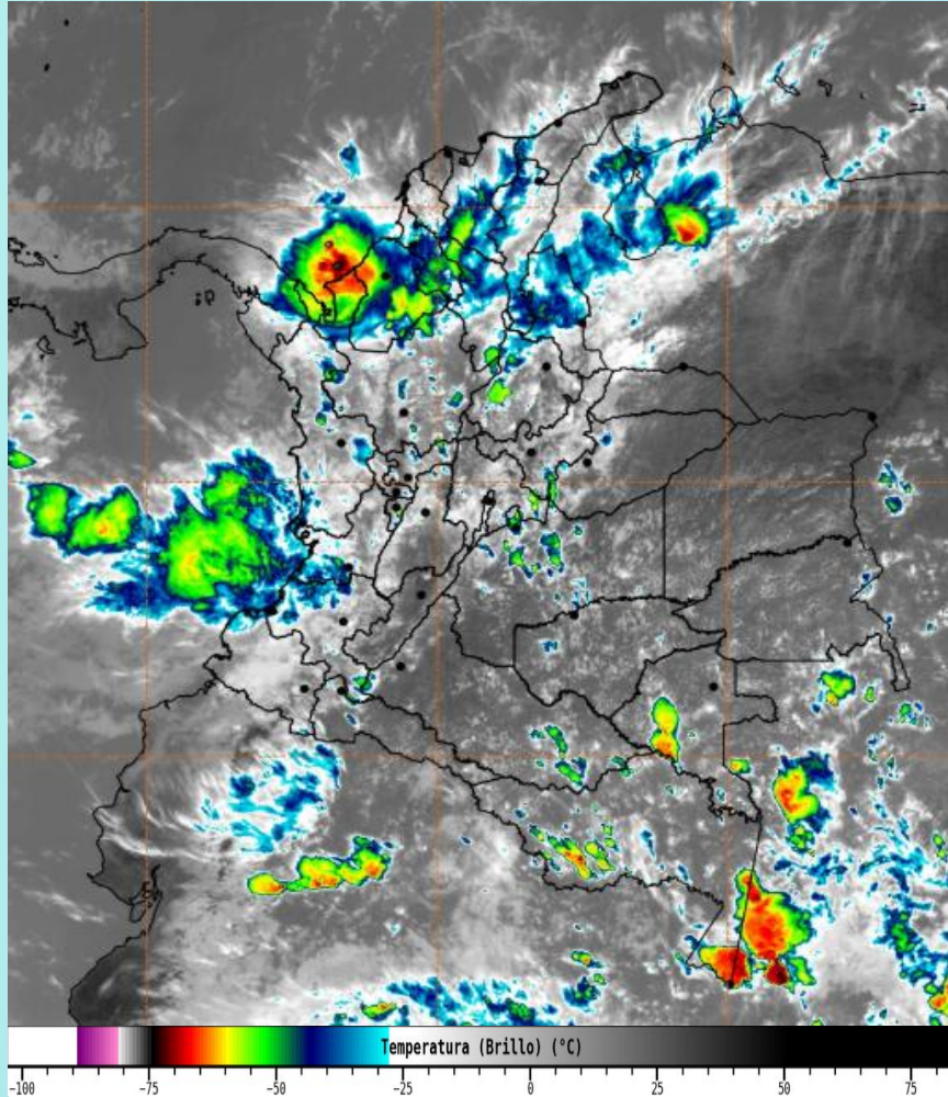
Imagen GOES 19 East Canal Infrarrojo, 5 de enero de 2026 - Hora 12:00 HLC. Fuente: https://bart.ideam.gov.co GOES 19
