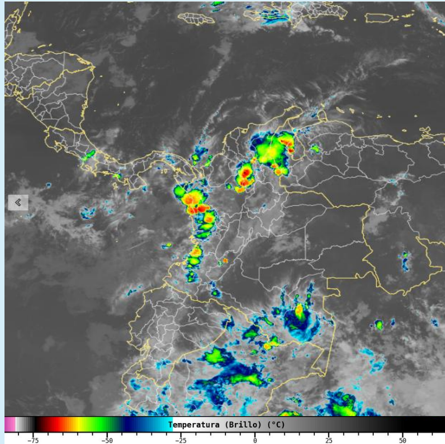
Imagen GOES 19 (East) Canal Infrarrojo 4 de enero de 2026– Hora 23:00 HLC Fuente: RAMMB - GOES 19
