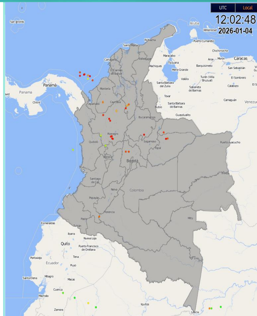
Descargas eléctricas en las últimas 3 horas. Hora 12:01 HLC Fuente: https://linetview.nowcast.de
