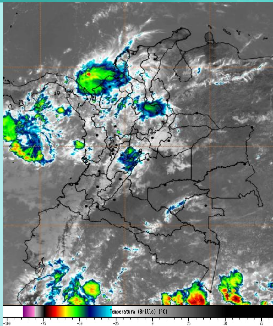
Imagen GOES 19 East Canal Infrarrojo, 4 de enero de 2026 - Hora 11:50 HLC. Fuente: https://bart.ideam.gov.co GOES 19
