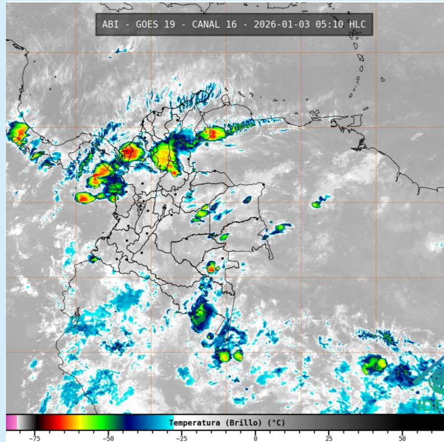
Imagen GOES 19 (East) Canal Infrarrojo 3 de enero de 2026– Hora 05:10 HLC Fuente: IDEAM – GOES 19
