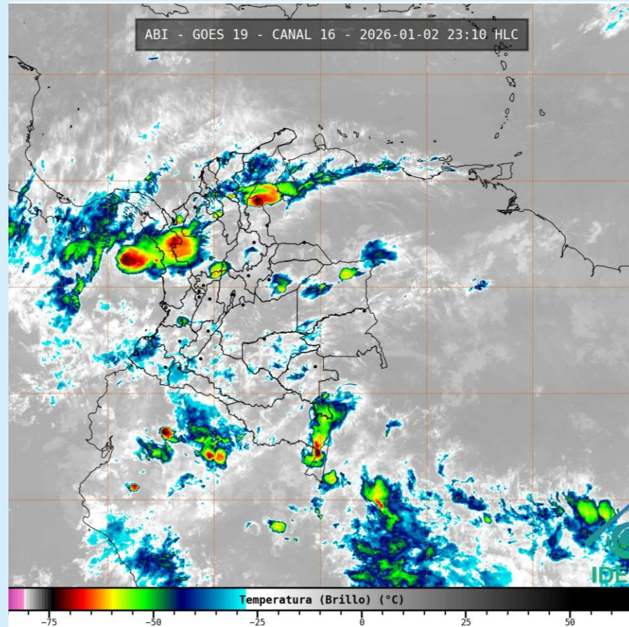
Imagen GOES 19 (East) Canal Infrarrojo 2 de enero de 2026– Hora 23:10 HLC Fuente: IDEAM – GOES 19
