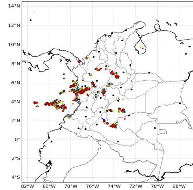
DESCARGAS ELÉCTRICAS GOES 19 MAPA NACIONAL PERIODO: 2026-01-02 04:05 - 2026-01-02 05:05 2026-01-02 04:05 - 2026-01-02 05:05 Elaborado por: Oficina del Servicio de Pronósticos y Alertas
