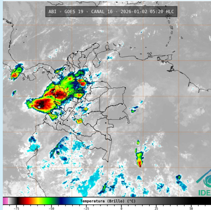
Imagen GOES 19 (East) Canal Infrarrojo 2 de enero de 2026– Hora 05:20 HLC Fuente: IDEAM – GOES 19
