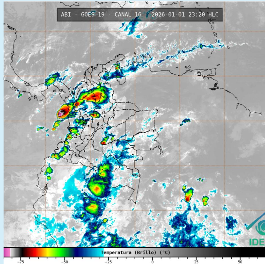
Imagen GOES 19 (East) Canal Infrarrojo 1 de enero de 2026– Hora 23:20 HLC Fuente: IDEAM – GOES 19
