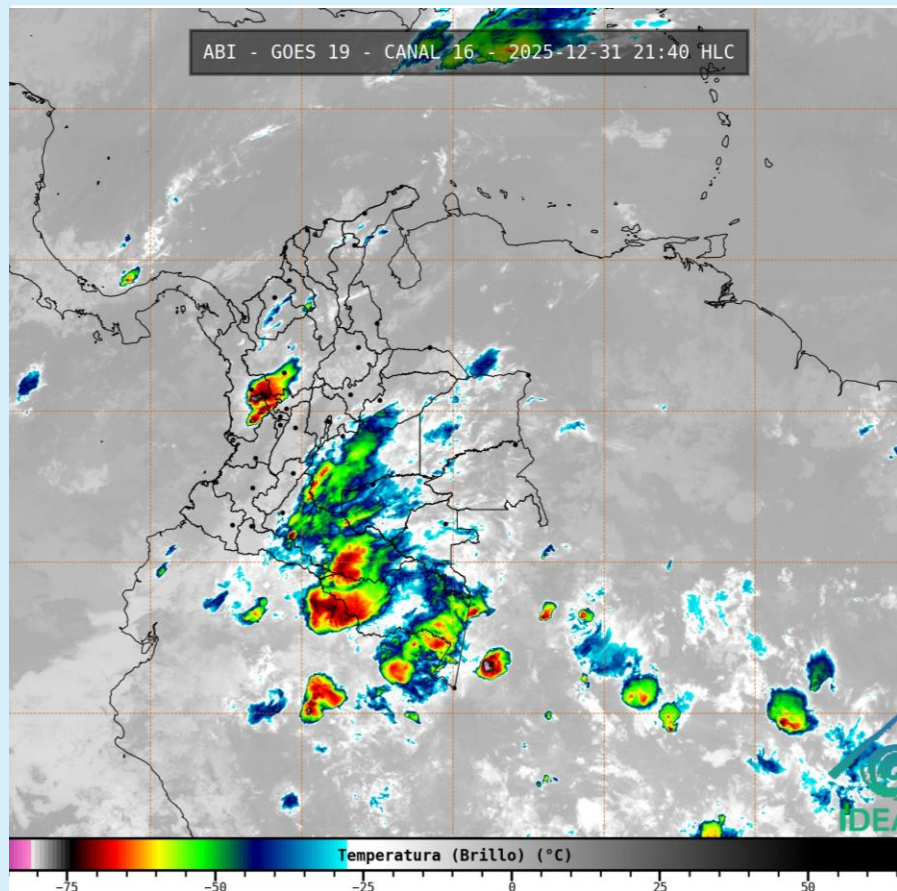
Imagen GOES 19 (East) Canal Infrarrojo 31 de diciembre de 2025– Hora 21:40 HLC Fuente: IDEAM – GOES 19
