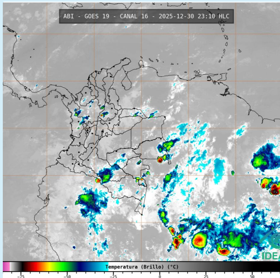
Imagen GOES 19 (East) Canal Infrarrojo 30 de diciembre de 2025– Hora 23:10 HLC Fuente: IDEAM – GOES 19
