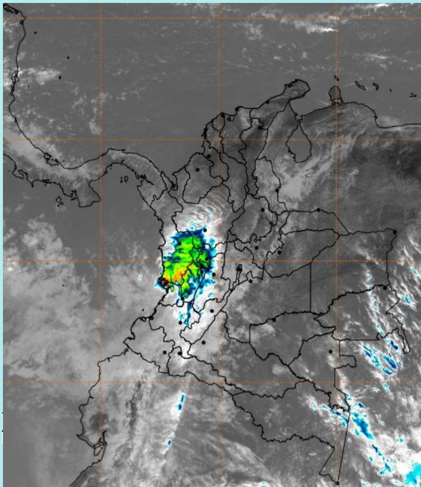
Imagen GOES 19 East Canal Infrarrojo, 25 de diciembre de 2025 - Hora 11:40 HLC. Fuente: https://bart.ideam.gov.co GOES 19
