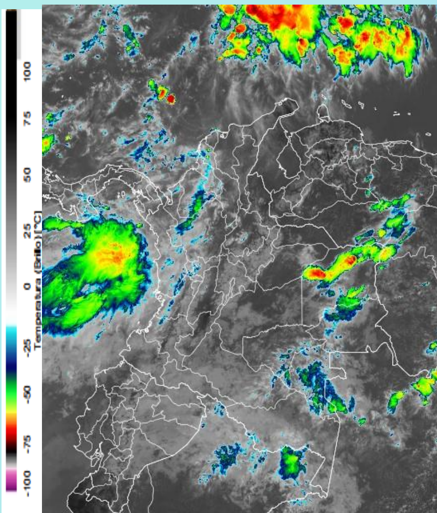
Imagen GOES East Canal Infrarrojo, 4 de julio de 2024 - Hora 11:40 HLC. Fuente: GOES 16
