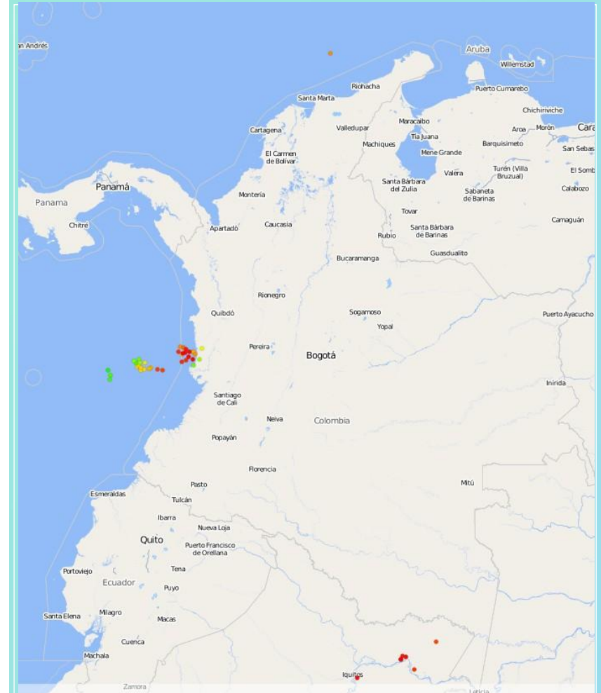
Descargas eléctricas en las últimas 3 horas. Hora 12:14 HLC Fuente: https://linetview.nowcast.de
