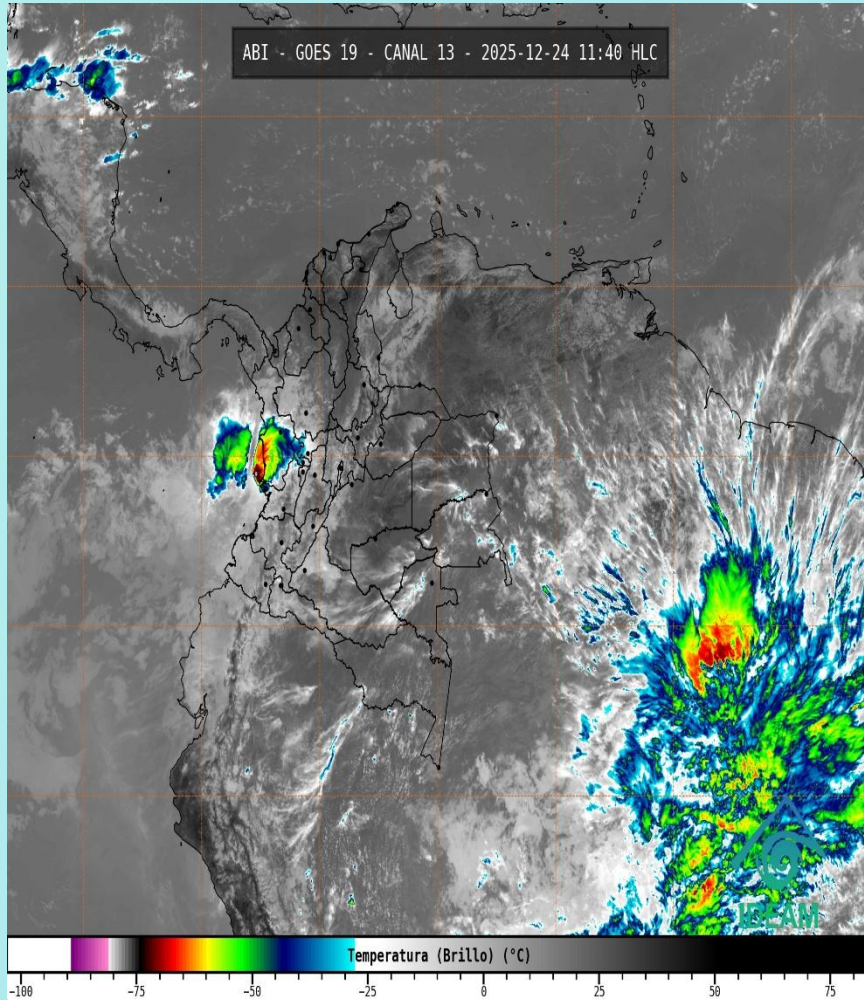
Imagen GOES 19 East Canal Infrarrojo, 24 de diciembre de 2025 - Hora 11:40 HLC. Fuente: https://bart.ideam.gov.co GOES 19
