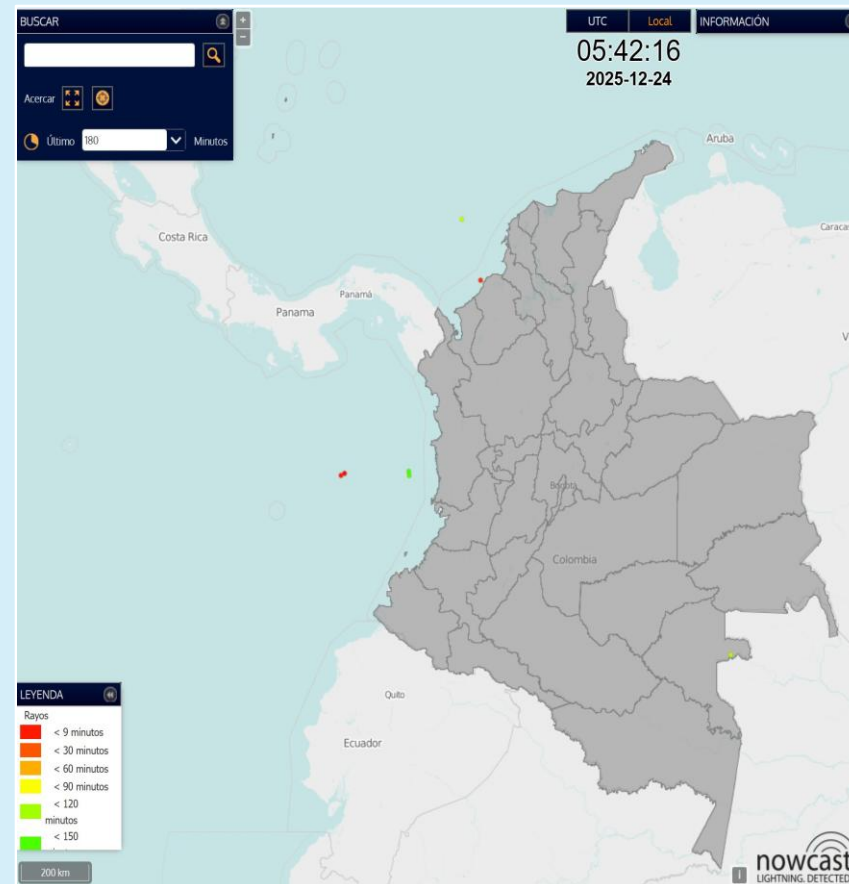
Descargas eléctricas (últimas horas) 24 de diciembre de 2025 – Hora 05:42 HLC Fuente: Keraunos
