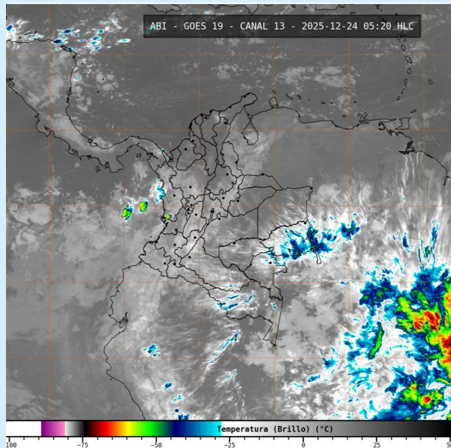
Imagen GOES 19 (East) Canal Infrarrojo 24 de diciembre de 2025 – Hora 05:20 HLC Fuente: IDEAM – GOES 19
