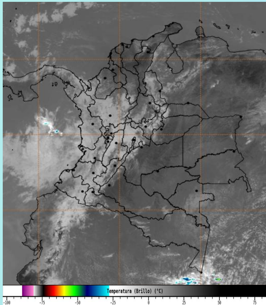
Imagen GOES 19 East Canal Infrarrojo, 22 de diciembre de 2025 - Hora 11:30 HLC. Fuente: https://bart.ideam.gov.co GOES 19
