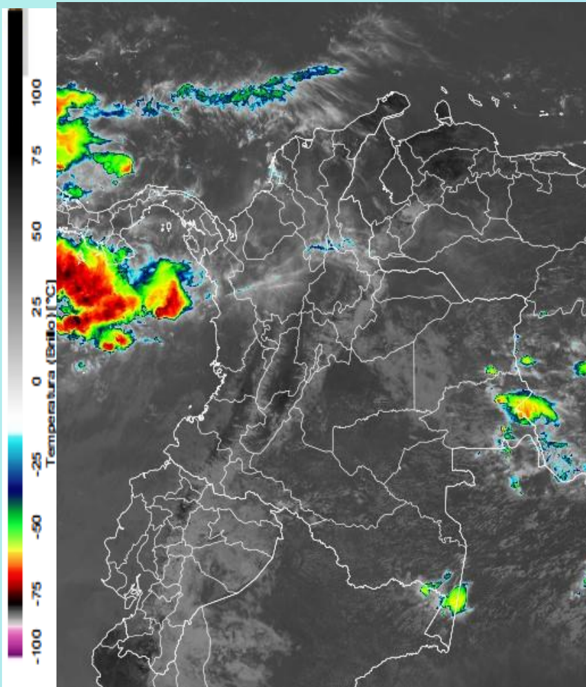
Imagen GOES East Canal Infrarrojo, 10 de julio de 2024 - Hora 11:40 HLC. Fuente: GOES 16
