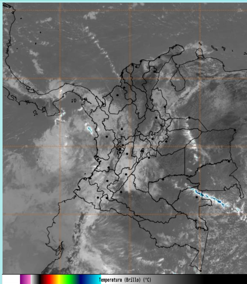
Imagen GOES 19 East Canal Infrarrojo, 21 de diciembre de 2025 - Hora 11:40 HLC. Fuente: https://bart.ideam.gov.co GOES 19
