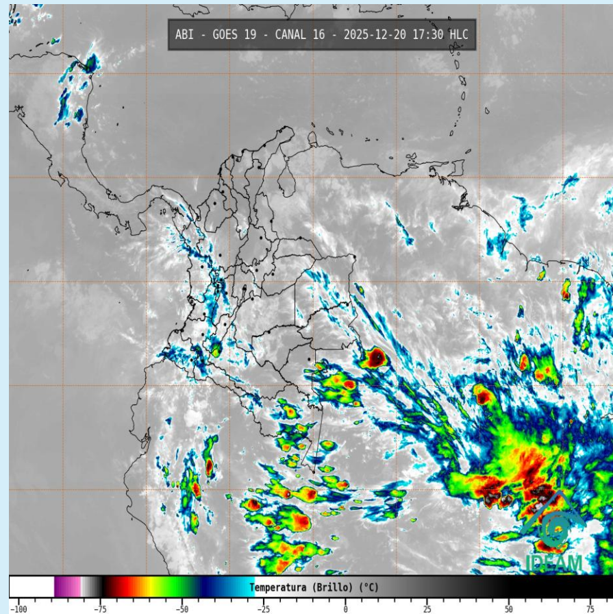
Imagen GOES 19 (East) Canal Infrarrojo 20 de diciembre de 2025– Hora 17:30 HLC Fuente: IDEAM – GOES 19
