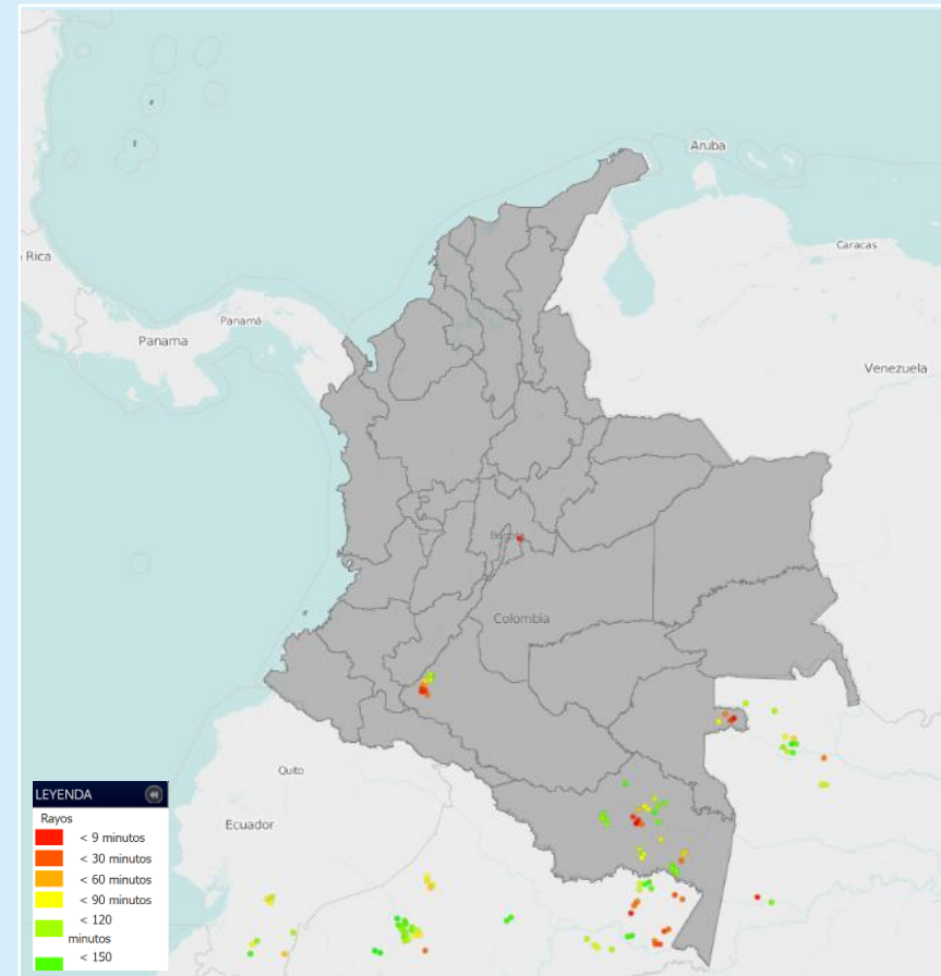
Descargas eléctricas (últimas horas) 20 de diciembre de 2025 – Hora 17:40 HLC Fuente: LINETVIEW KERAUNOS
