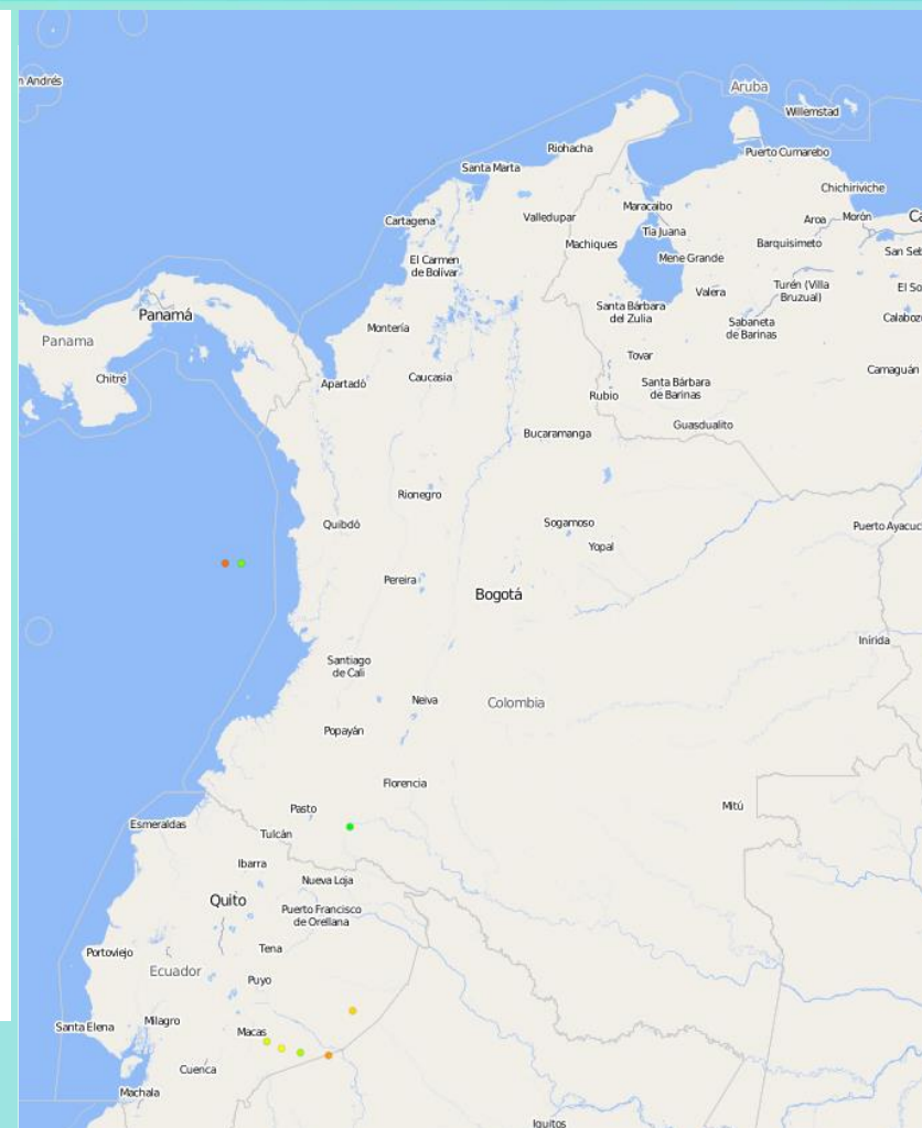
Descargas eléctricas en las últimas 3 horas. Hora 12:10 HLC Fuente: https://linetview.nowcast.de
