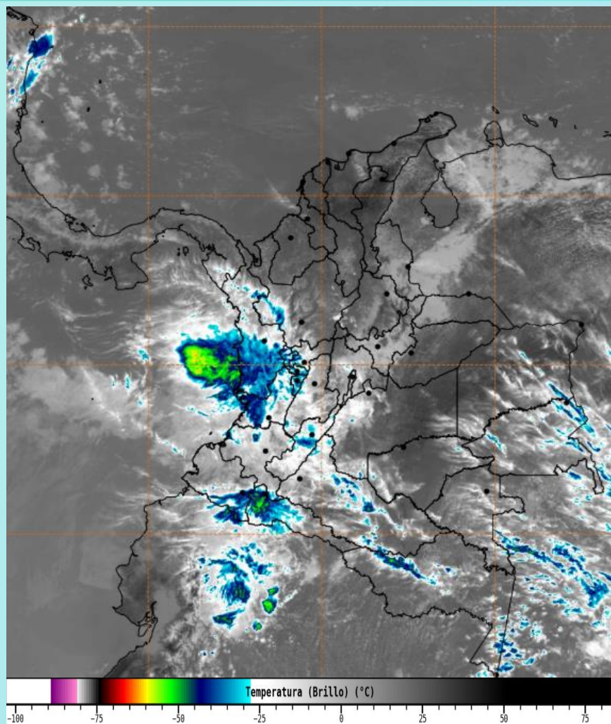
Imagen GOES 19 East Canal Infrarrojo, 20 de diciembre de 2025 - Hora 11:50 HLC. Fuente: https://bart.ideam.gov.co GOES 19
