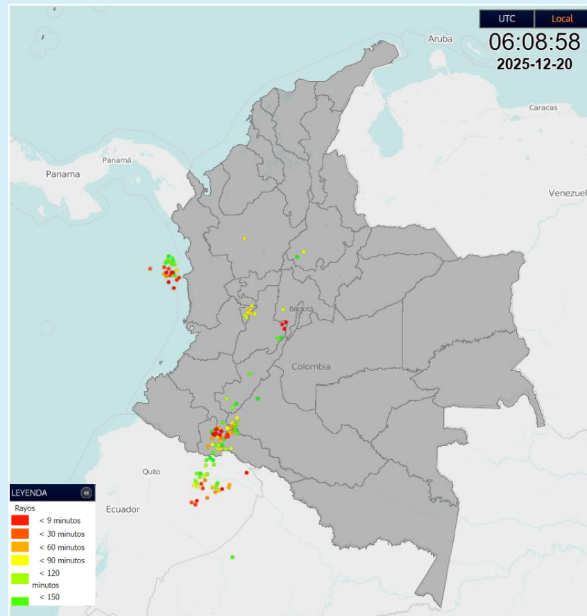
Descargas eléctricas (últimas horas) 20 de diciembre de 2025 – Hora 06:08 HLC Fuente: LINETVIEW KERAUNOS
