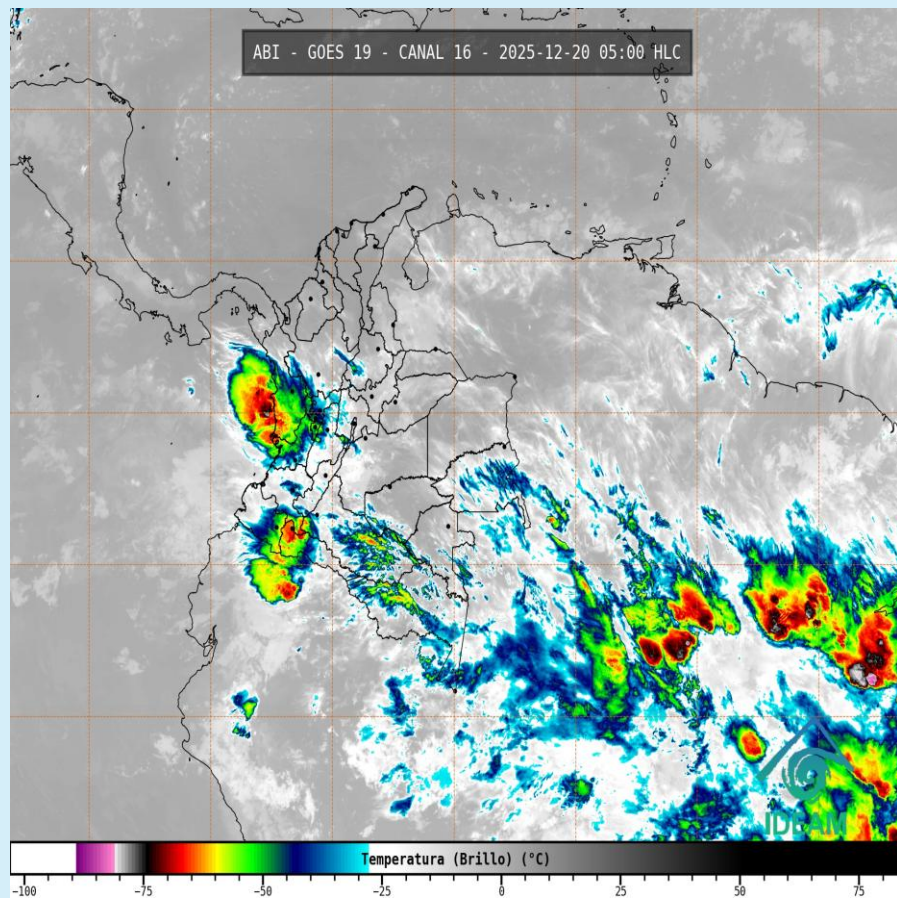
Imagen GOES 19 (East) Canal Infrarrojo 20 de diciembre de 2025 – Hora 05:00 HLC Fuente: IDEAM – GOES 19
