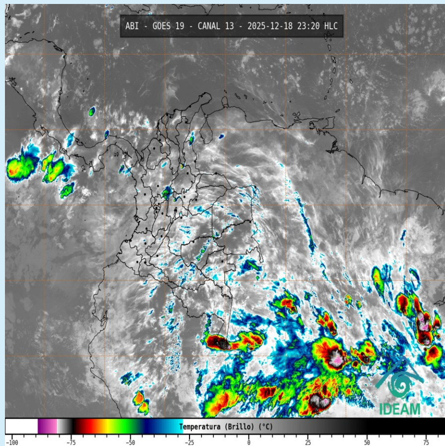
Imagen GOES 19 (East) Canal Infrarrojo 18 de diciembre de 2025– Hora 23:20 HLC Fuente: IDEAM – GOES 19
