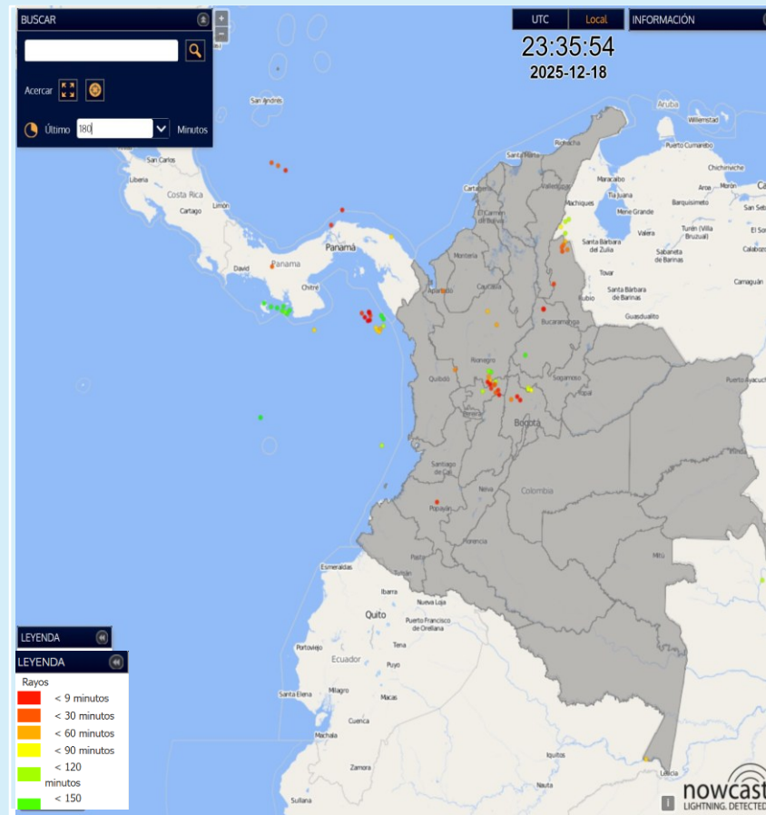
Descargas eléctricas (últimas horas) 18 de diciembre de 2025 – Hora 23:35 HLC Fuente: LINETVIEW KERAUNOS
