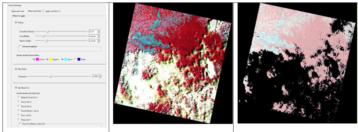
Figura 5. Plug-in Cloud Masking, enmascaramiento de nubes y sombras de nubes.
