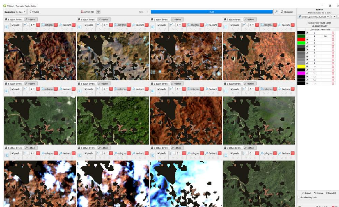
Figura 10. Edición cambios por deforestación zona de Paramillo año 2023
