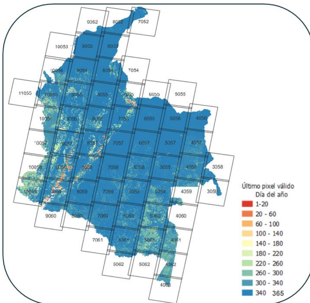
Figura 8. Mosaico de jday-last-pixel de 2023. Imágenes Landsat.
