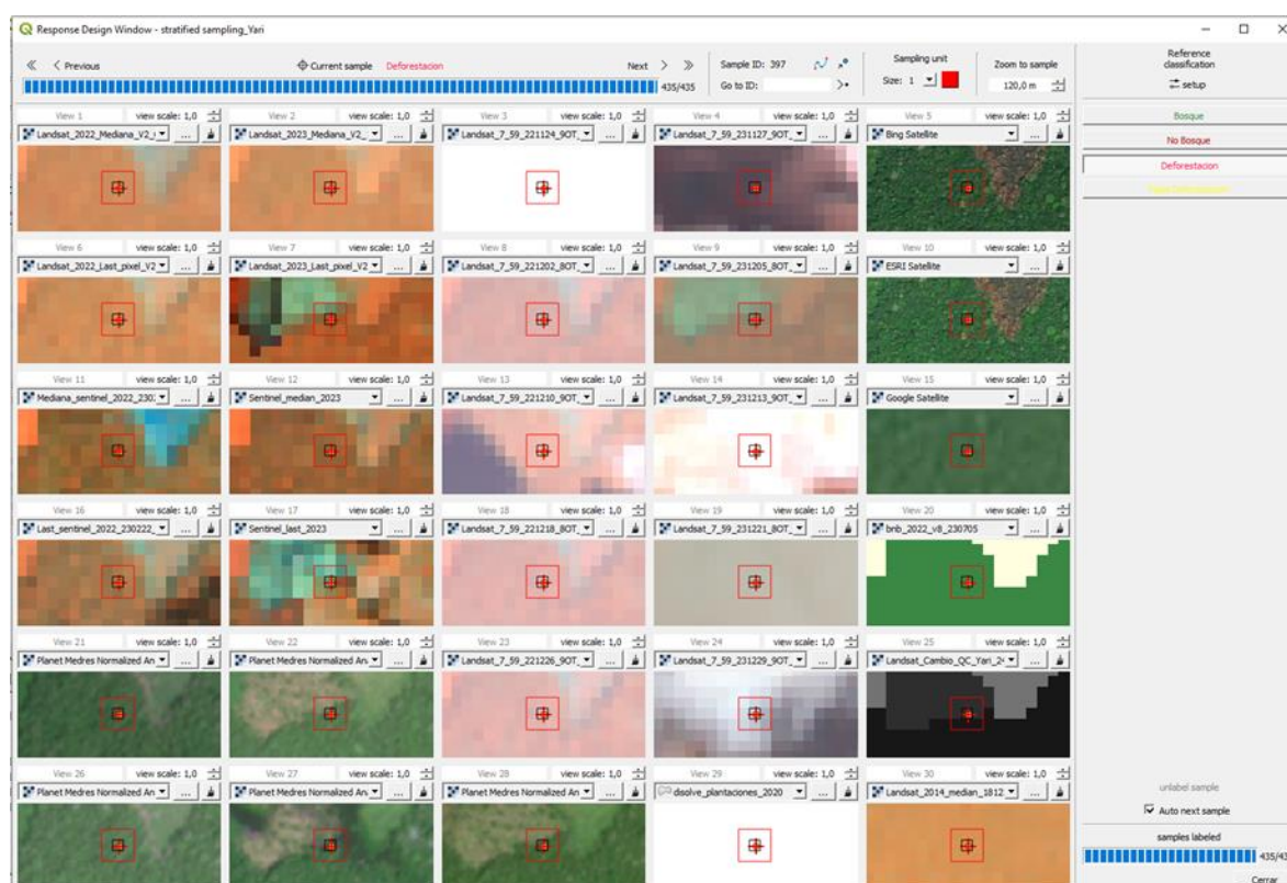
Figura 14. Clasificación de las muestras utilizando AcATaMa.
