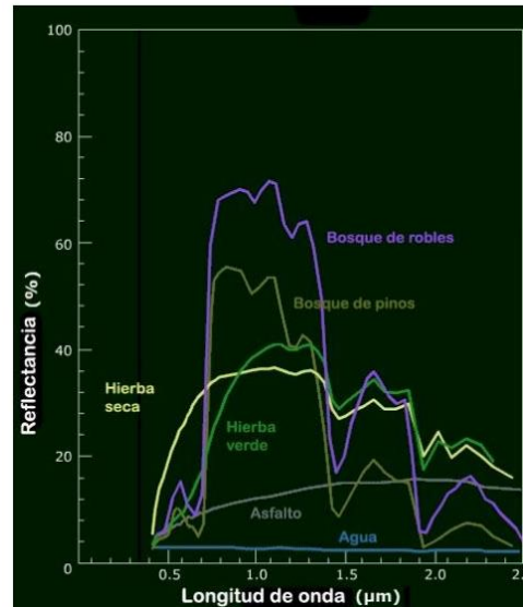
Figura 3. Firmas o respuesta espectral para diferentes elementos de la superficie de la tierra.
