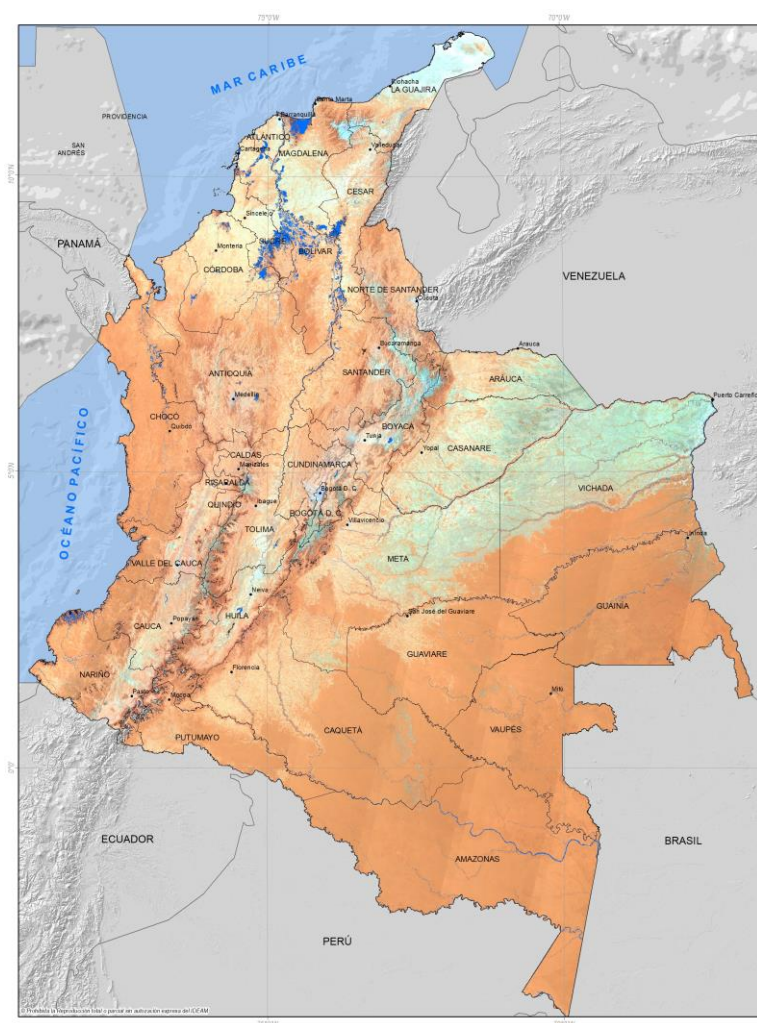
Figura 9. Mosaico de Mediana estadística del año 2023.
