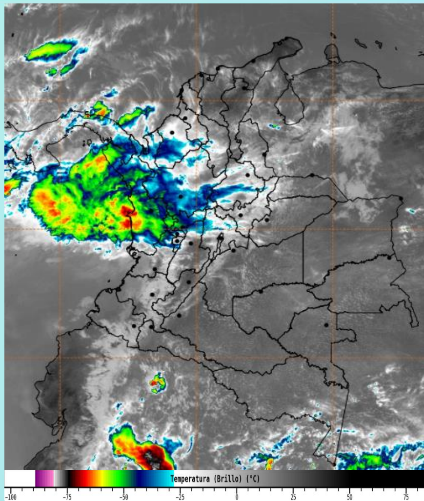
Imagen GOES 19 East Canal Infrarrojo, 12 de diciembre de 2025 - Hora 12:00 HLC. Fuente: https://bart.ideam.gov.co GOES 19
