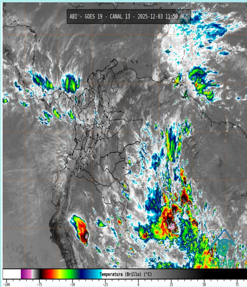
Imagen GOES 19 East Canal Infrarrojo, 3 de diciembre de 2025 - Hora 11:50 HLC. Fuente: IDEAM GOES 19
