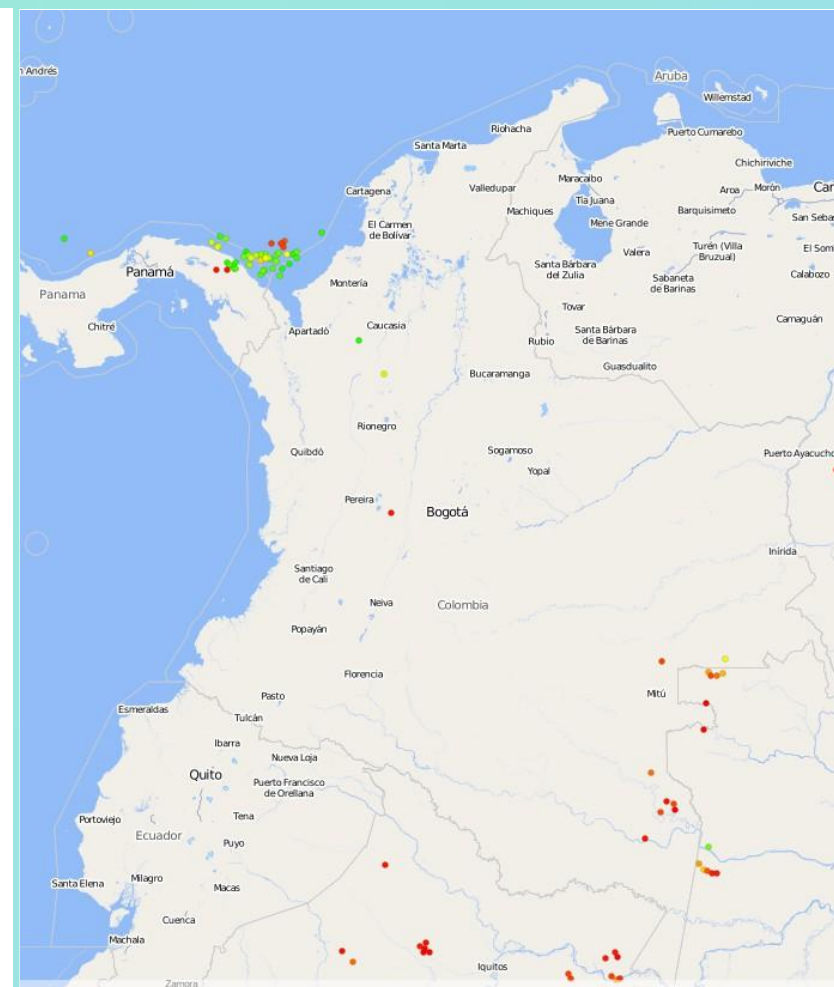
Descargas eléctricas en las últimas tres horas. Hora 12:11 HLC Fuente: https://linetview.nowcast.de/linetview/pages/index.html
