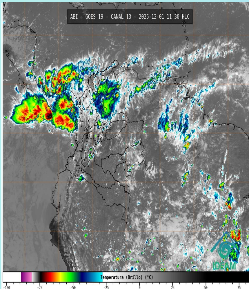
Imagen GOES 19 East Canal Infrarrojo, 1 de diciembre de 2025 - Hora 11:30 HLC. Fuente: IDEAM GOES 19
