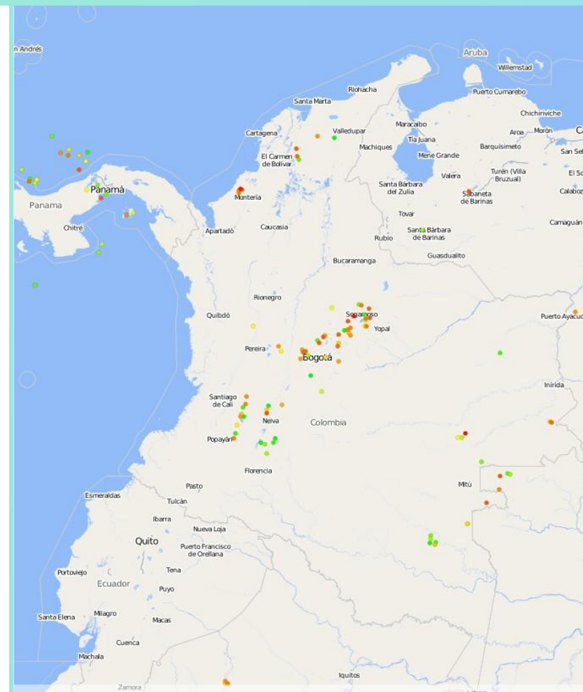
Descargas eléctricas en los últimos treinta minutos. Hora 12:20 HLC Fuente: https://linetview.nowcast.de/linetview/pages/index.html
