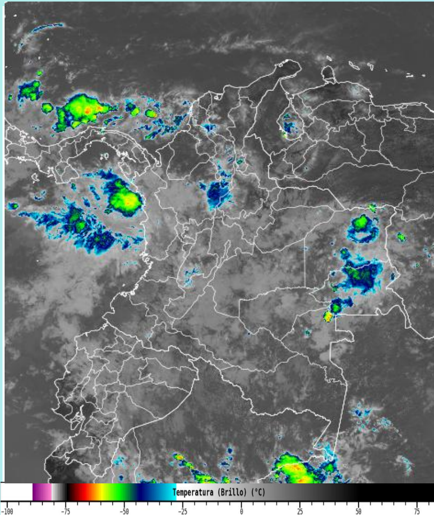
Imagen GOES 19 East Canal Infrarrojo, 14 de noviembre de 2025 - Hora 12:20 HLC. Fuente: IDEAM
