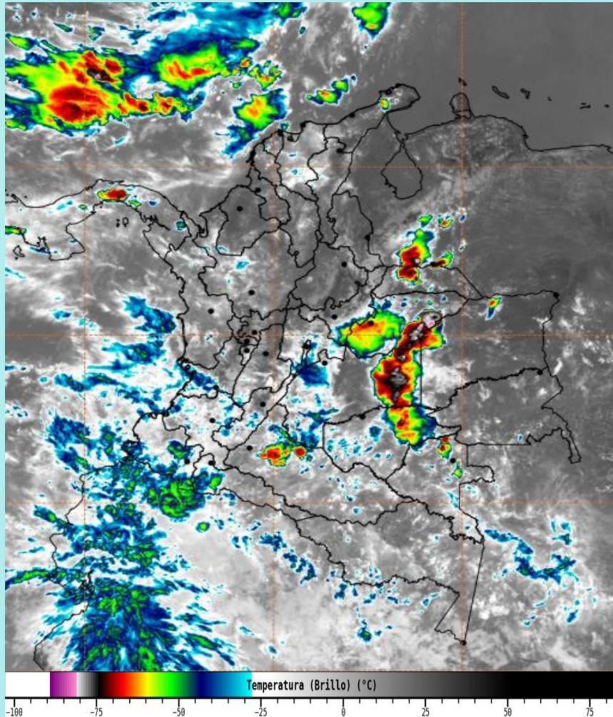
Imagen GOES 19 East Canal Infrarrojo, 29 de octubre de 2025 - Hora 12:00 HLC. IDEAM – GOES 19
