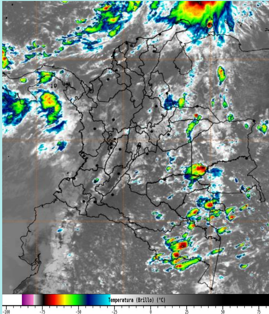
Imagen GOES 19 East Canal Infrarrojo, 25 de octubre de 2025 - Hora 12:20 HLC. IDEAM – GOES 19
