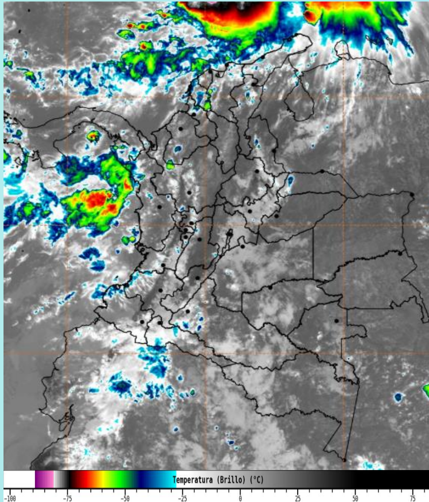
Imagen GOES 19 East Canal Infrarrojo, 24 de octubre de 2025 - Hora 11:50 HLC. IDEAM – GOES 19
