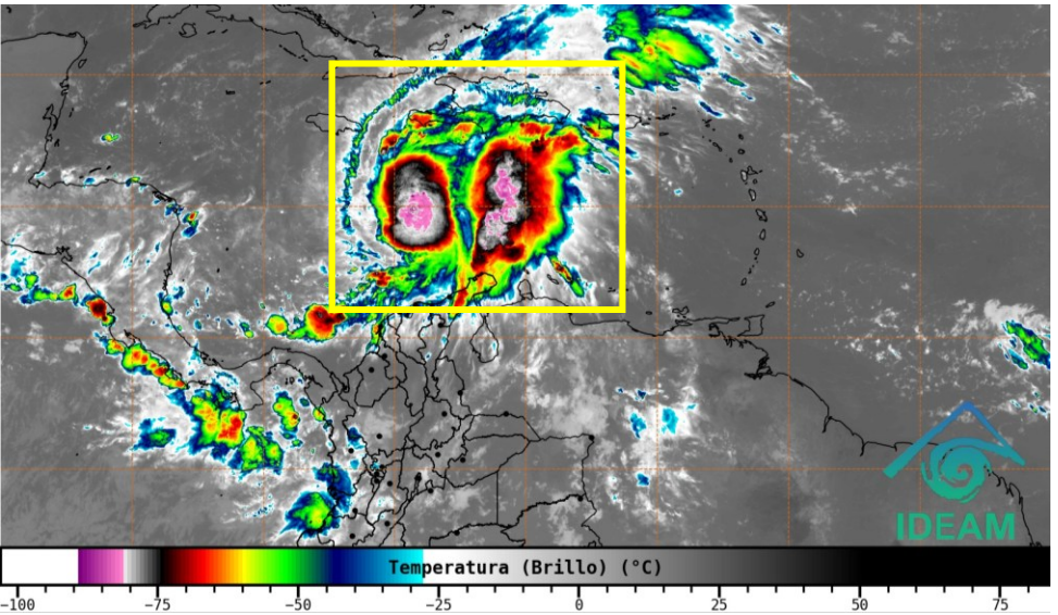
Imagen Satelital GOES -19. Canal Infrarrojo. octubre 24 de 2025, 07:20 HLC Fuente: GOES-IDEAM
