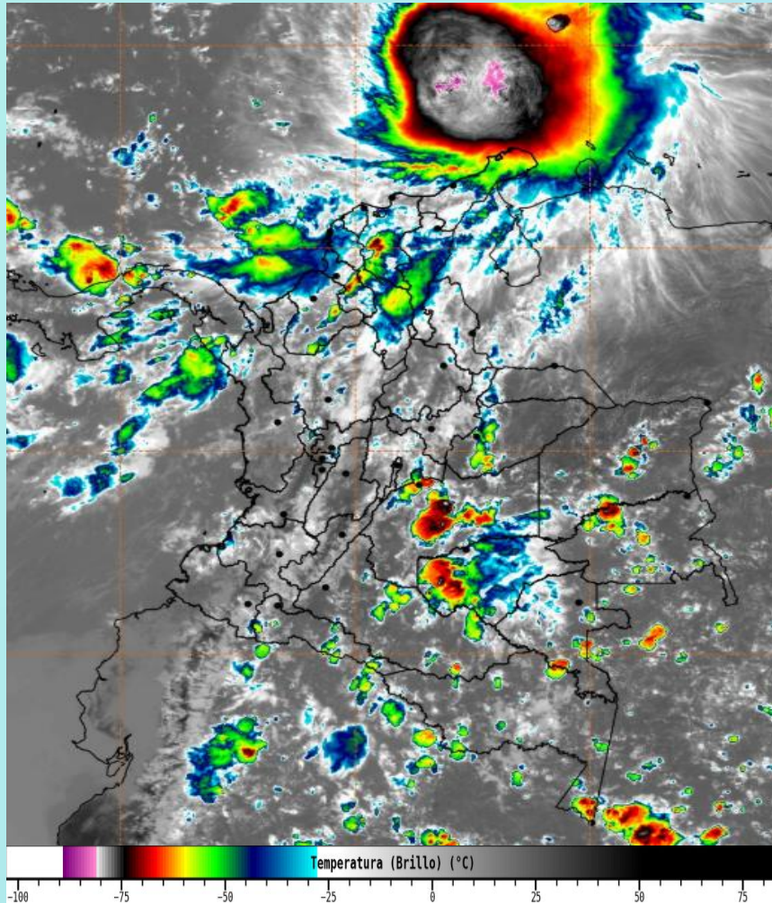
Imagen GOES 19 East Canal Infrarrojo, 22 de octubre de 2025 - Hora 12:00 HLC. IDEAM – GOES 19
