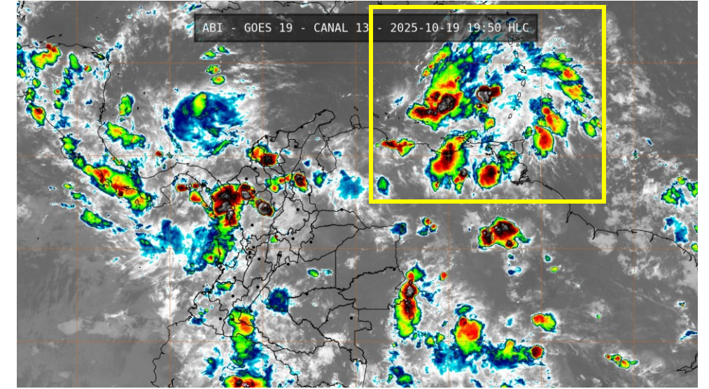
Imagen Satelital GOES -19. Canal Infrarrojo. octubre 19 de 2025, 19:50 HLC Fuente: GOES-IDEAM
