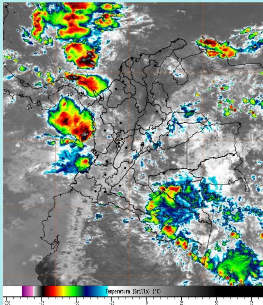
Imagen GOES 19 East Canal Infrarrojo, 19 de octubre de 2025 - Hora 11:50 HLC. IDEAM – GOES 19
