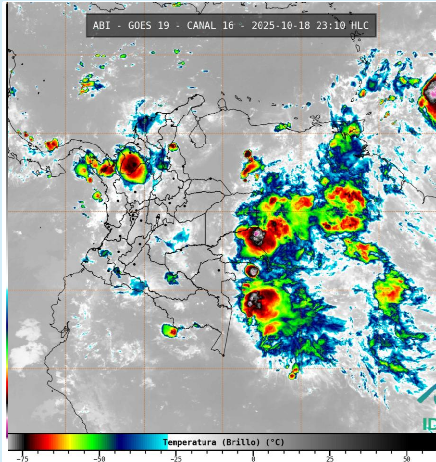
Imagen GOES 19 (East) Canal Infrarrojo 18 de octubre de 2025 – Hora 23:10 HLC Fuente: IDEAM – GOES 19
