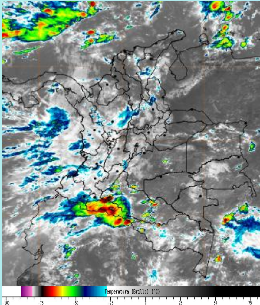
Imagen GOES 19 East Canal Infrarrojo, 12 de octubre de 2025 - Hora 11:30 HLC. IDEAM – GOES 19
